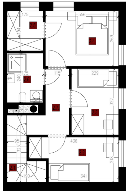
PIĘTRO zestawienie pomieszczeń ( Lokal 1 )
